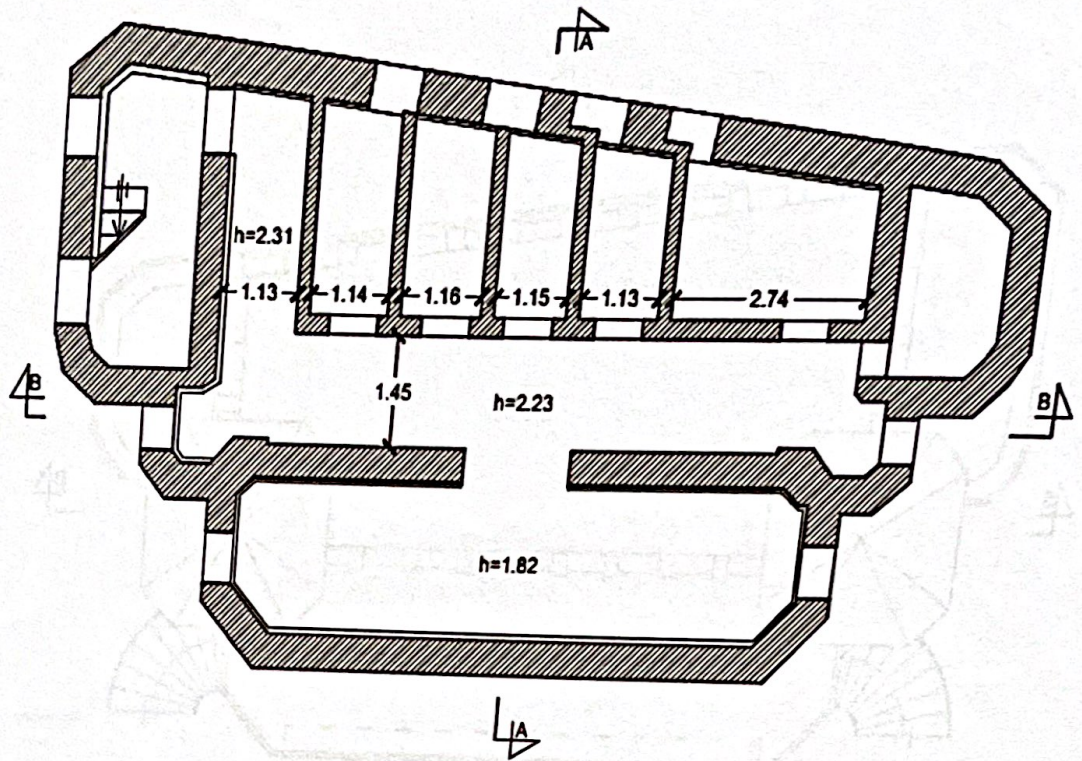
PIANTA ALLA QUOTA DEL PIANO CANTINATO
